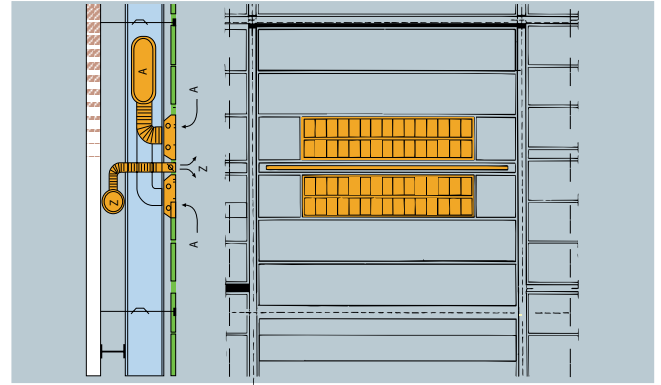
Bild 1: Schnitt u. Unteransicht der Decke mit Zu- u. Abluftführung
