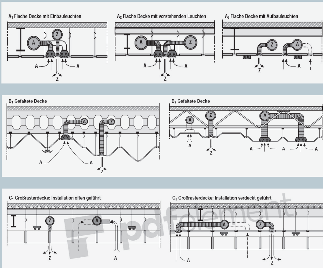
Bild 3: Ausbildungsformen integrierter Deckensysteme (vgl. Tabelle 1)
